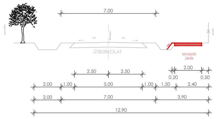
B-B metszet
